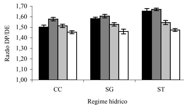
FIGURA 21. Relação diâmetro polar equatorial em mudas de café cv Catuaí IAC 99 submetidas a: CC (capacidade de campo), SG (suspensão gradativa da irrigação) e ST (suspensão total da irrigação) e pulverizadas com diferentes soluções após dose dias de estresse: controle (■); H 2 O 2 (■); ácido ascórbico duas horas após o H 2 O 2 (■) e ácido ascórbico (□). As barras representam o erro padrão da média de 50 repetições. UFLA, Lavras, MG, 2007.
