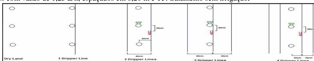
Figura 1 – Distribuição dos tubo gotejadores nas linhas de café, Fazenda Experimental de Varginha.
