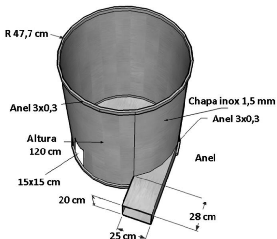
Figura 26. Detalhes internos do ciclone com entrada tangencial inferior e porta de limpeza.
