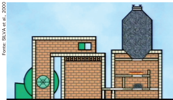
Fonte: SILVA et al., 2000 Figura 29. Corte longitudinal da fornalha mostrando a opção por construir um duto (30cm x30 cm) em alvenaria para ligar o ciclone ao ventilador.
