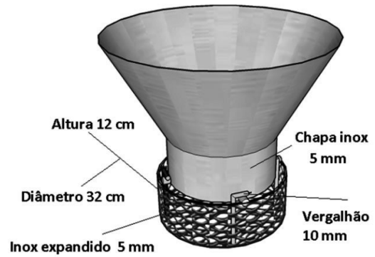
Figura 23. Depósito de carvão ou briquete e detalhe da grelha suspensa e removível.
