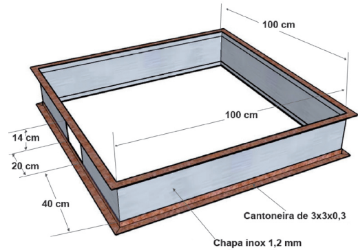
Figura 14. Módulo 2 ou base metálica para a construção do cinzeiro (observe a abertura para retirada das cinzas).
