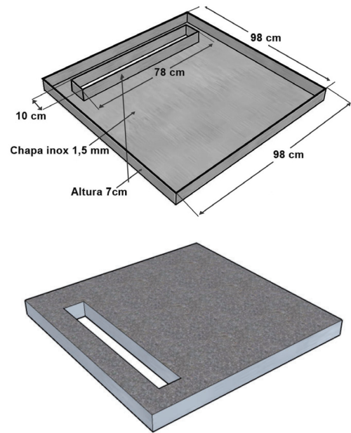
Figura 4. Forma e laje concretada para separar a base e o cinzeiro da fornalha.
