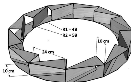
Figura 28. Coroa metálica para auxiliar a montagem do ciclone (pode ser substituída por tijolos comuns).
