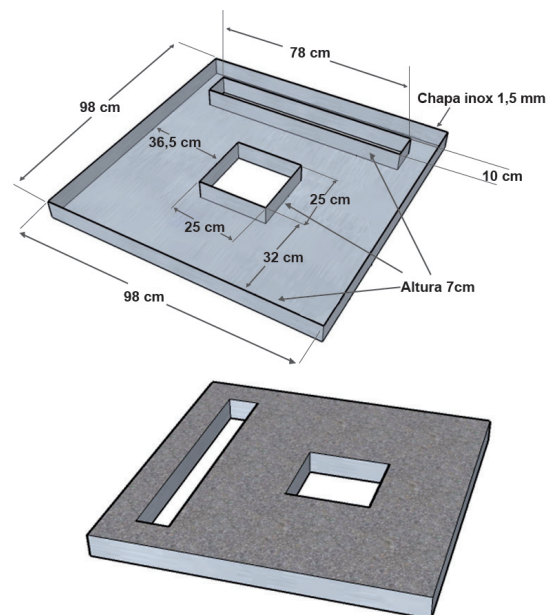
Figura 5. Forma e laje concretada para separar o cinzeiro da câmara de combustão.
