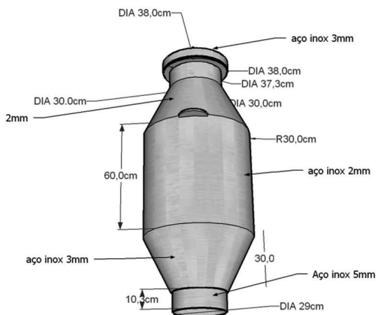
Figura 23. Depósito de carvão ou briquete e detalhe da grelha suspensa e removível.
