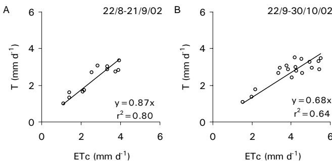
Figura 2. Relação entre a transpiração máxima (T) e a evapotranspiração do cafezal em dois períodos subsequentes: (A) sem a presença de vegetação ativa na entrelinha; (B) entrelinha ocupada pela vegetação rasteira.
