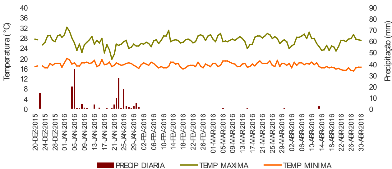
Gráfico 13 – Temperaturas (Máxima e Mínima) da Estação Meteorológica Automática - Piatã - Bahia (BA) - Precipitação do modelo COSMO nas coordenadas de Piatã-BA
