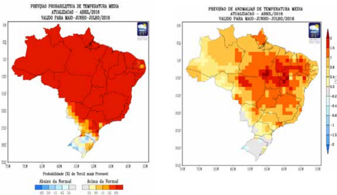
Figura 9 – Previsão climática de temperatura média (probabilidades e anomalias) de maio, junho e julho/2016
