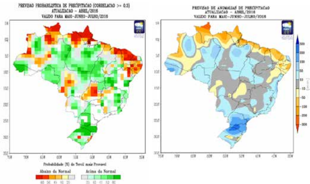
Figura 8 – Previsão climática de precipitação (probabilidades e anomalias) de maio, junho e julho/2016
