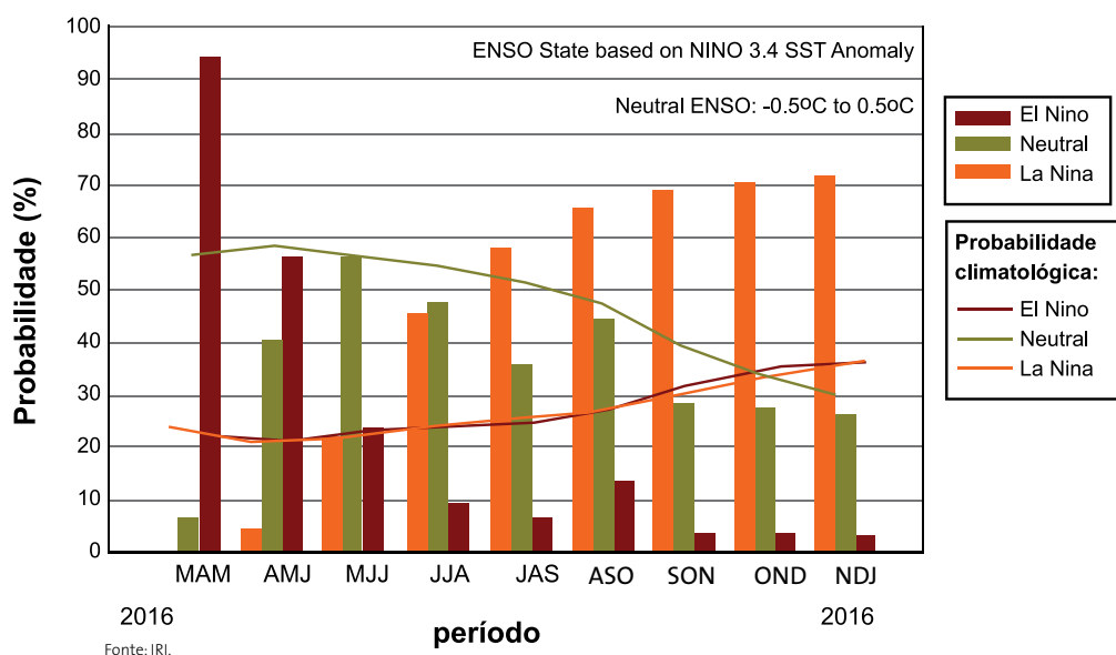
Gráfico 3 - Previsão probabilística de El Niño
