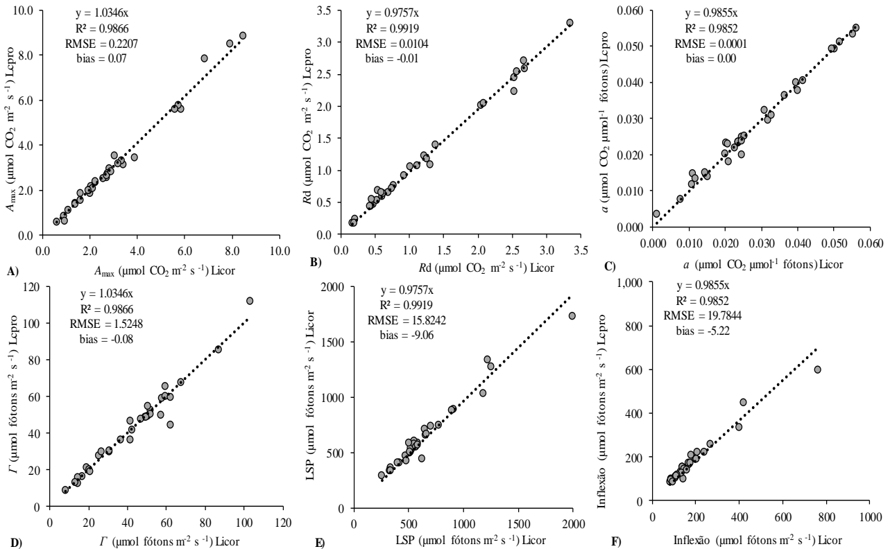
Figura 2. Comparação entre Licor 6400 e LC-pro através de regressão linear para os parâmetros calculados a partir de curvas A/PAR. Medições realizadas em folhas de cafeeiros, 40 dias após encerramento de injeção de \text{CO}_2 adicional no prévio experimento FACE de longa duração: A) fotossíntese máxima ( A_{\max} , \mu\text{mol m}^{-2} \text{s}^{-1} ), B) respiração no escuro ( R_d , \mu\text{mol m}^{-2} \text{s}^{-1} ), C) eficiência quântica aparente ( \alpha , \mu\text{mol } \mu\text{mol}^{-1} ), D) ponto de compensação de luz ( \Gamma , \mu\text{mol fótons m}^{-2} \text{s}^{-1} ), E) ponto de saturação de luz (LSP, \mu\text{mol fótons m}^{-2} \text{s}^{-1} ) e F) ponto de inflexão ( \mu\text{mol fótons m}^{-2} \text{s}^{-1} ).
