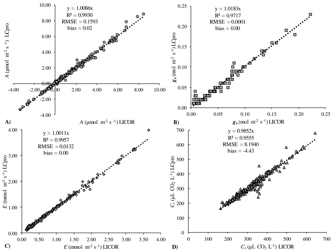
Figura1. Comparação de medições realizadas com Licor 6400 e LC-pro através de regressão linear para os valores de trocas gasosas de folhas de cafeeiros. Medições foram realizadas 40 dias após encerramento de injeção de \text{CO}_2 adicional no prévio experimento FACE de longa duração: A) fotossíntese ( A , \mu\text{mol m}^{-2} \text{ s}^{-1} ), B) condutância estomática ( g_s , \text{mol m}^{-2} \text{ s}^{-1} ), C) transpiração foliar ( E , \text{mmol m}^{-2} \text{ s}^{-1} ) e D) concentração interna de \text{CO}_2 ( C_i , \mu\text{mol mol}^{-1} ).
