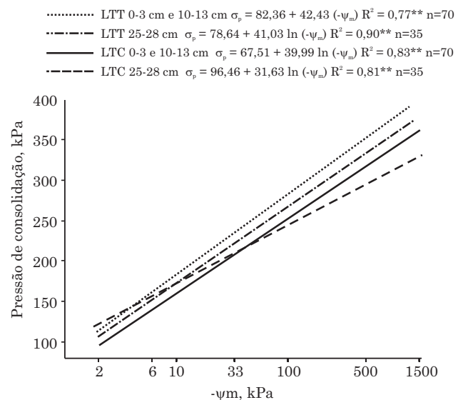
Figura 2. Modelo de capacidade de suporte de carga em função do potencial matricial ( -\psi_m ) em um Latossolo Vermelho-Amarelo (LVA) para a linha de tráfego do trator (LTT) e linha de tráfego da colhedora (LTC), em três camadas sob a cultura do café.
